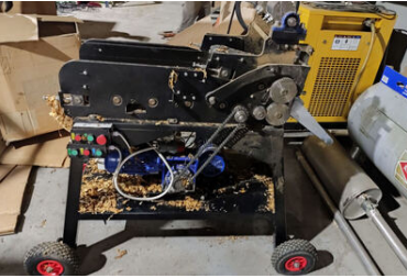
Zabezpieczona maszyna do produkcji nielegalnych papierosów
