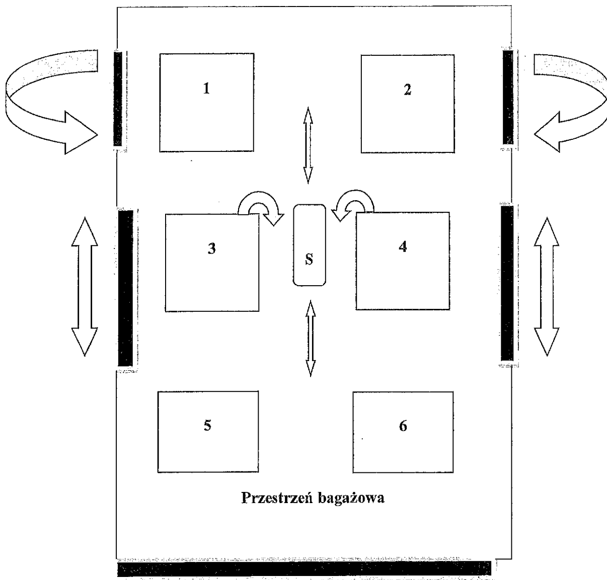
Układ drzwi i siedzeń – vide rozdział V pn. „Część pasażerska” niniejszego OPZ. S – stół składany z możliwością przesuwu wzdłuż osi podłużnej pojazdu
