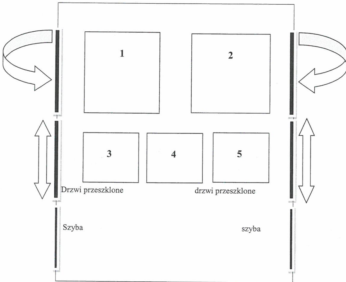
Układ drzwi i siedzeń vide V część pasażerska punkt 1 i 2 (Drzwi przestrzeni bagażowej unoszone, przeszkłone).
